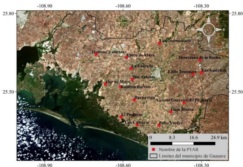
Figura 2. Localización de las 16 PTAR con fosa séptica+wetland para el tratamiento de las aguas residuales generadas en localidades rurales.
